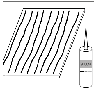
Silikonraupen vertikal auftragen (1cm vom Rand entfernt und 6 cm Abstand zwischen den einzelnen Silikonraupen) Apply beads of silicone vertically (1cm from the edge and with 6cm-spaces between the individual beads).
