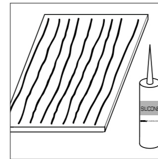
Silikonraupen vertikal auftragen Apply beads of silicone vertically
